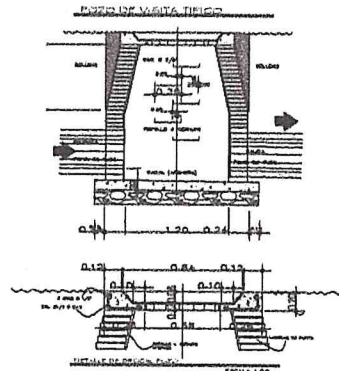
PARA TUBERIAS DE UNA RED DE ALICANTARILLADO EN BARRAS NORMALES
